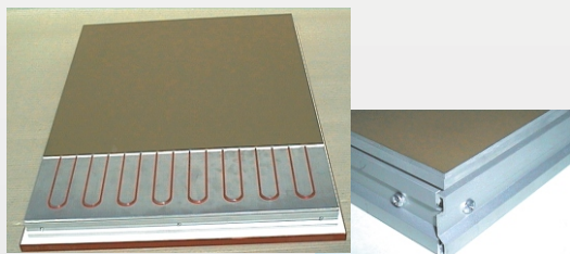
Schnitt durch eine Elektro-Kombi-Heizplatte ( Teilansicht ) und Detail Kantenschutz.
