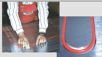
ELKOM Sicherheits-Heizleiter (Patent DBP 4239568)
